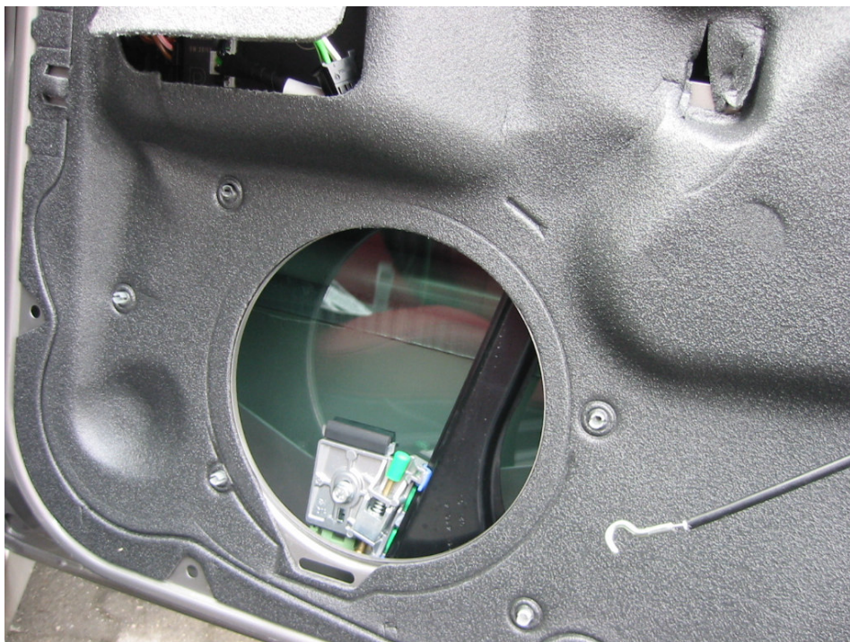
Der ausgebaute Tieftöner - Platz bis zur Scheibenmechanik ca 20 mm Zwischen Innenverkleidung und dem Blech sind es noch mal ca 40 mm ( eigentlich ist dann noch Spielraum – aber das wird dann Detailarbeit ) Durchmesser im Blech ~ 180 mm
